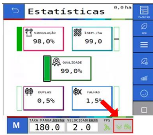
Figura 131 - Indicação do status do sensor de levante
