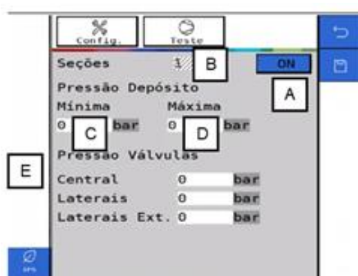
Figura 55 - Tela de configuração de molas pneumáticas
