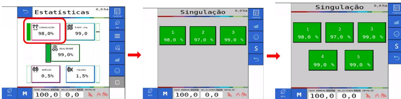
Figura 122 - Linhas e funções de visualização da tela de plantio ISOBUS
